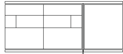
3 Ante da 60 3 60mm doors 1 Vano a giorno 1 Storage unit
