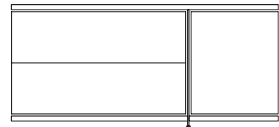
2 Ante Ribalta da 120 2 120mm tilting doors 1 Anta da 60 1 60mm door
